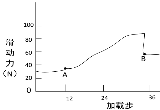
图1 滑坡过程滑动力监测曲线
