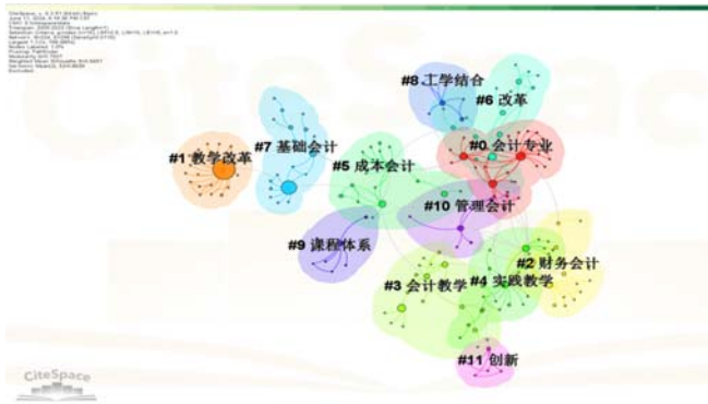
图2 关键词聚类情况
