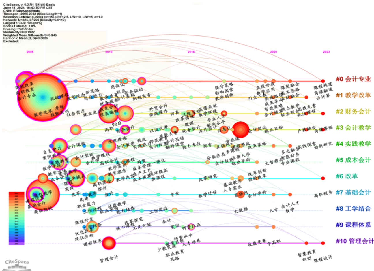
图4 关键词时间线演进图谱
